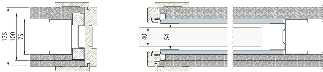
Opbouw 3 | Met 2 lagen gips: Totale wanddikte 100 mm - Metalstud 75 mm - Afwerkpakket 125mm
