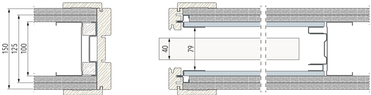
Opbouw 7 | Met 2 lagen gips: Totale wanddikte 150 mm - Metalstud 100 mm - Afwerkpakket 150mm
