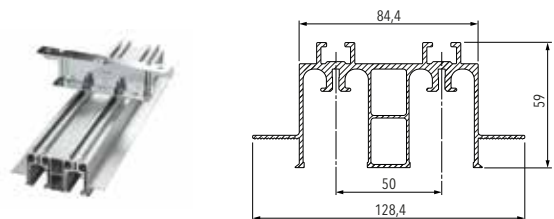
DUBBEL
