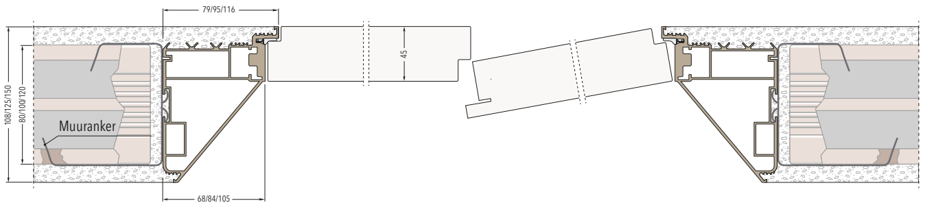
PULL - DEUR RECHTS, LINKS VAST
