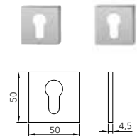
PROFIELCILINDER SLOTT (exclusief cilinder)
