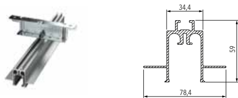
ENKEL
