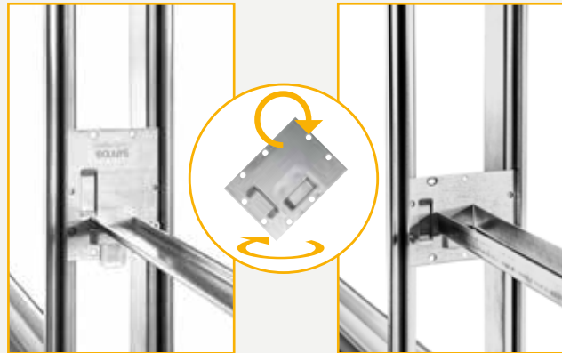
Afstandhouder: TH 100 mm
