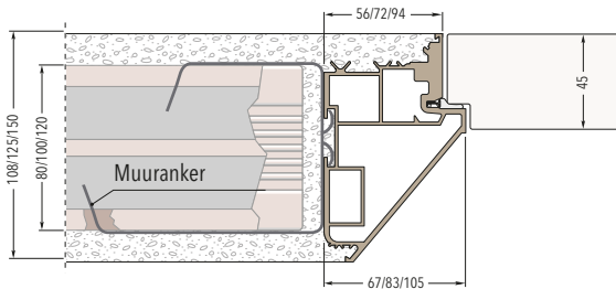
NAAR BINNENDRAAIENDE DEUR / PUSH VERSIE
