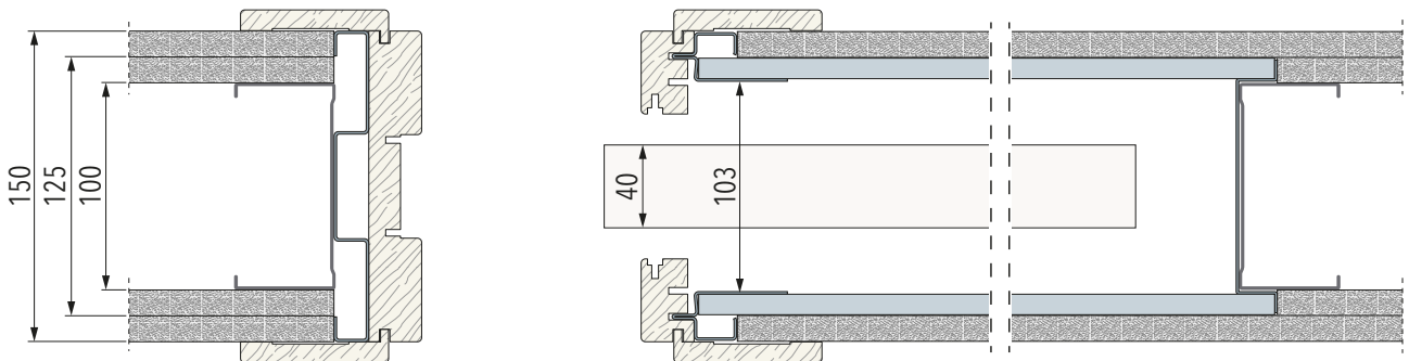
Opbouw 8 | Met 1 laag gips op de cassette: Totale wanddikte 150 mm - Metalstud 100 mm - Afwerkpakket 150mm
