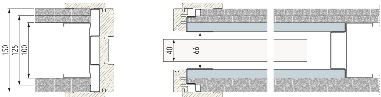
Opbouw 9 | Met 2 lagen gips: Totale wanddikte 150 mm - Metalstud 100 mm - Afwerkpakket 150mm
