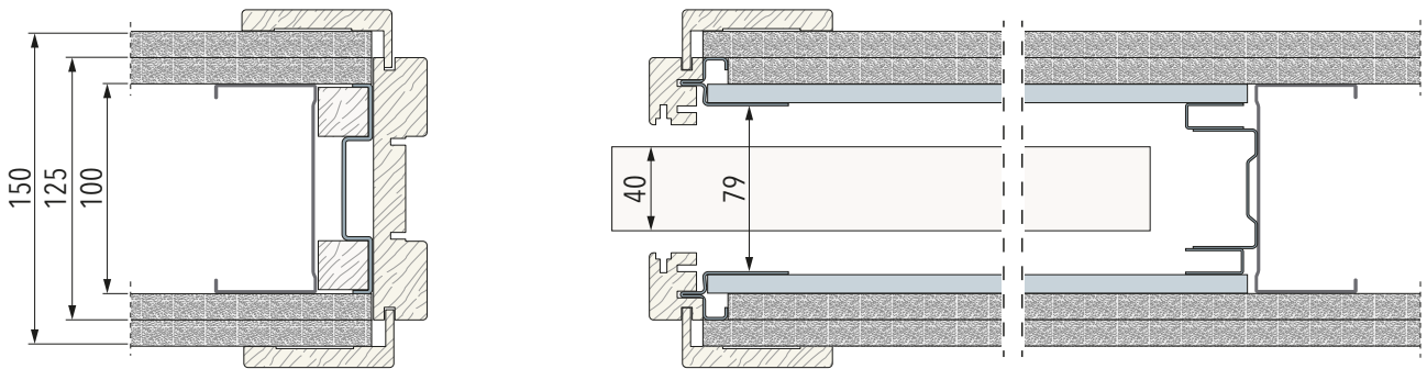
Opbouw 6 | Met 2 lagen gips: Totale wanddikte 150 mm - Metalstud 100 mm - Afwerkpakket 125mm
