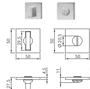
VRIJ/BEZET SLOTT
