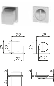
VRIJ/BEZET SLOTT
