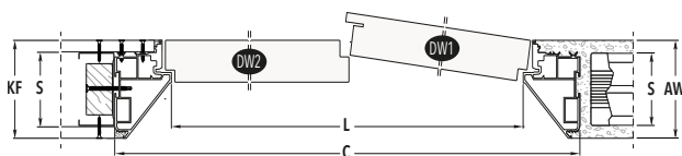
PUSH VERSIE
