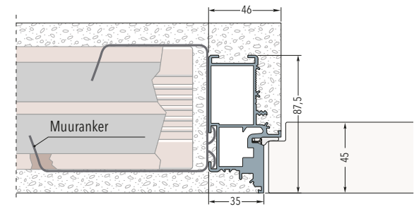
NAAR BUITENDRAAIENDE DEUR / PULL VERSIE
