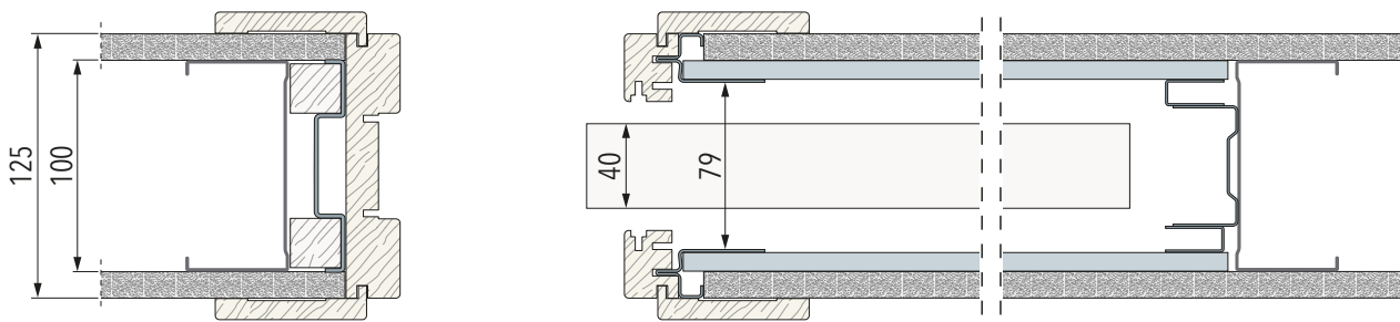
Opbouw 5 | Met 1 laag gips: Totale wanddikte 125 mm - Metalstud 100 mm - Afwerkpakket 125mm
