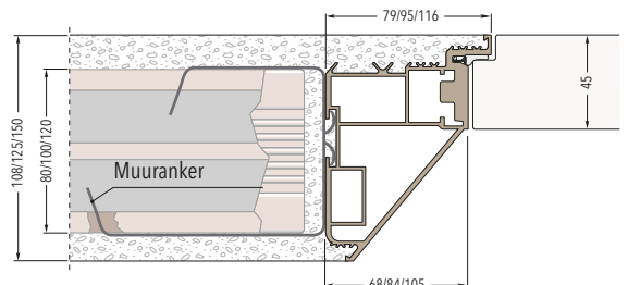
NAAR BUITENDRAAIENDE DEUR / PULL VERSIE
