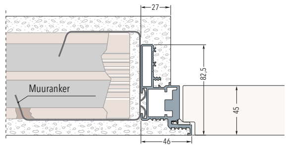
NAAR BINNENDRAAIENDE DEUR / PUSH VERSIE
