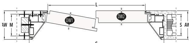
PULL VERSIE
