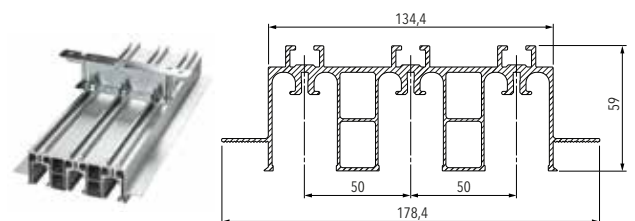
DRIEDUBBEL
