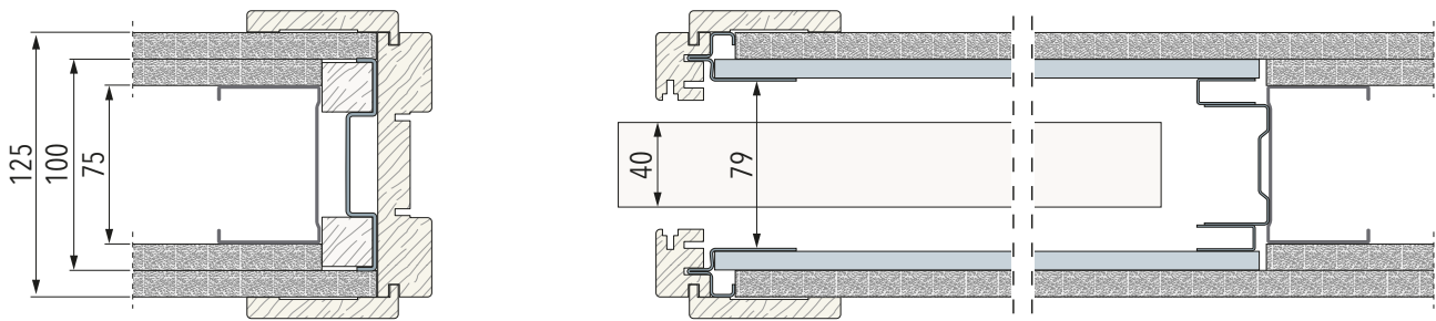
Opbouw 4 | Met 1 laag gips op de cassette: Totale wanddikte 125 mm - Metalstud 75 mm - Afwerkpakket 125mm
